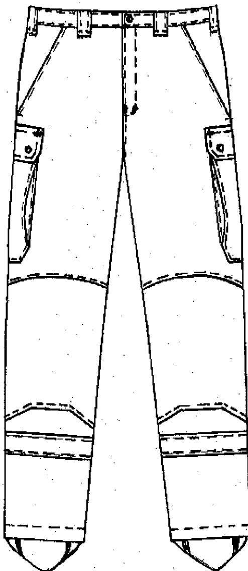
Скица 3. Предна част
